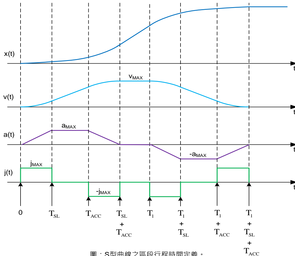
圖：S型曲線之區段行程時間定義。
