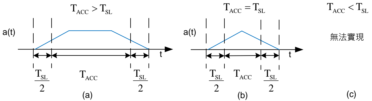
圖：S型曲線之行程時間定義。
