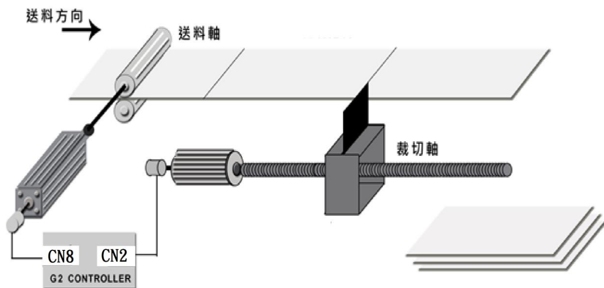
圖 5.3 追剪示意圖
