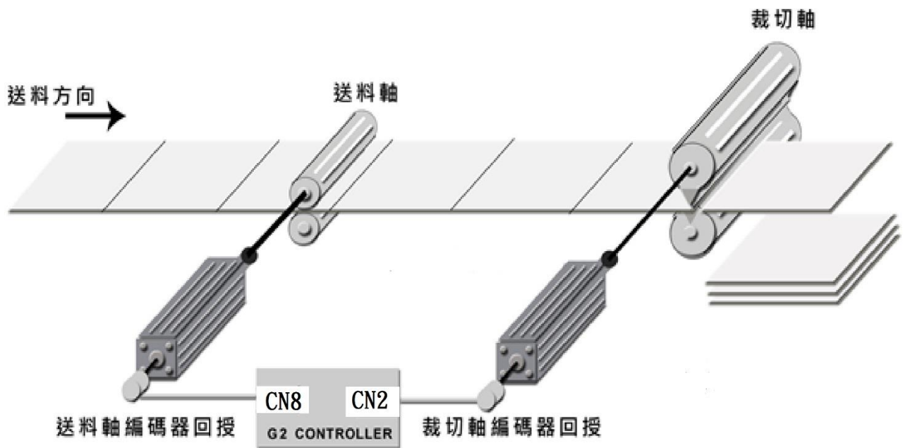
飛剪示意圖
